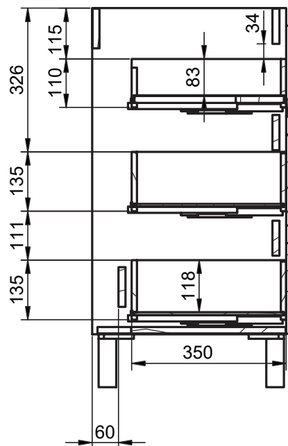
B-B ( 1 : 10 )
